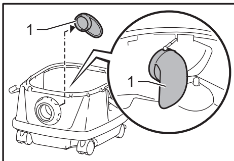
► 1. Rubber holder
